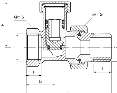
DN15
