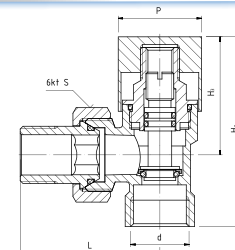
ZAWÓR GRZEJNIKOWY ODCINAJĄCY
