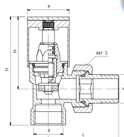
ZAWÓR GRZEJNIKOWY ZASILAJĄCY
